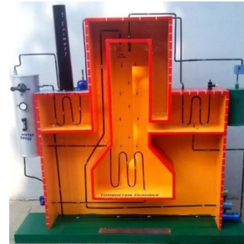
B. Velox Boiler
